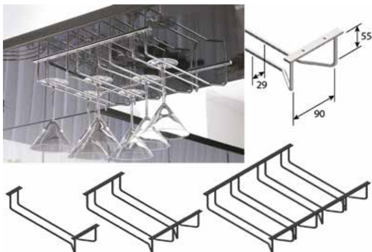
Support pour verres - montage au plafond
