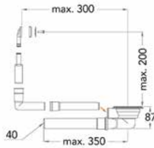
Crépine Space Saver avec trop plein rectangulaire
