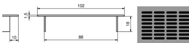
Grilles d'aération avec hauteur 102 mm - grands trous ovales - grands trous ovales: 30 x 6 mm
